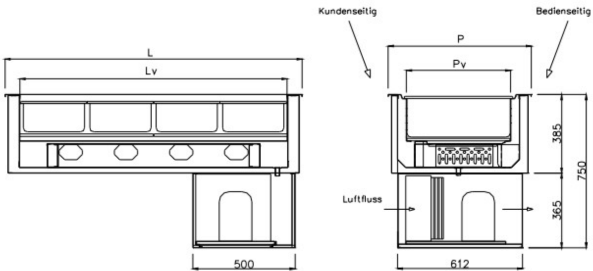
Sicht Bedienseitig
