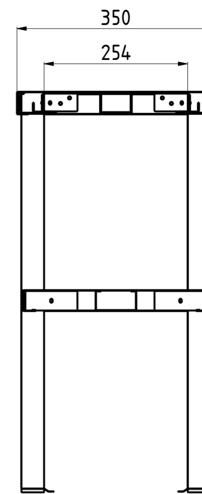
A-A
