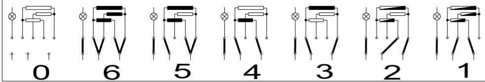
SCHEMA COLLEGAMENTO COMMUTATORE
