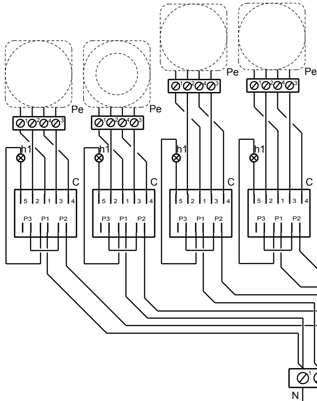
SCHEMA COLLEGAMENTO COMMUTATORE
